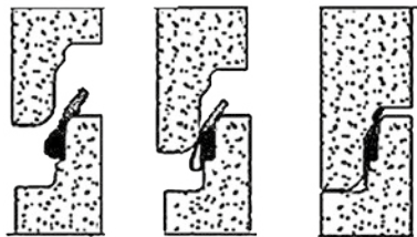
Prinsippskisse kumskjøt
